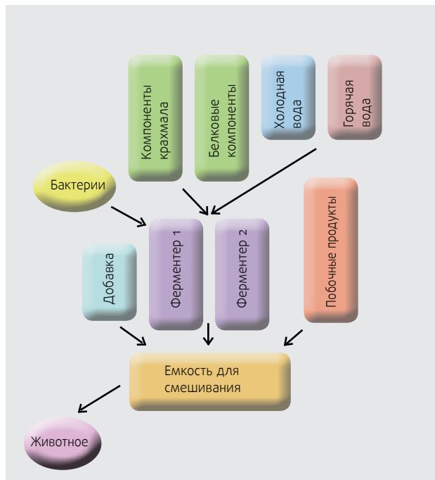
Смешивание в ферментере
