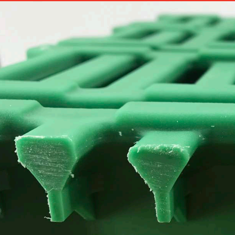
断面図：円錐形のため洗浄時に残留物がたまりません
