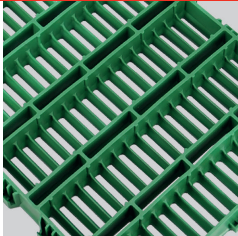
ダブルバー構造により、希望する理想的なサイズに容易にカットできます。
